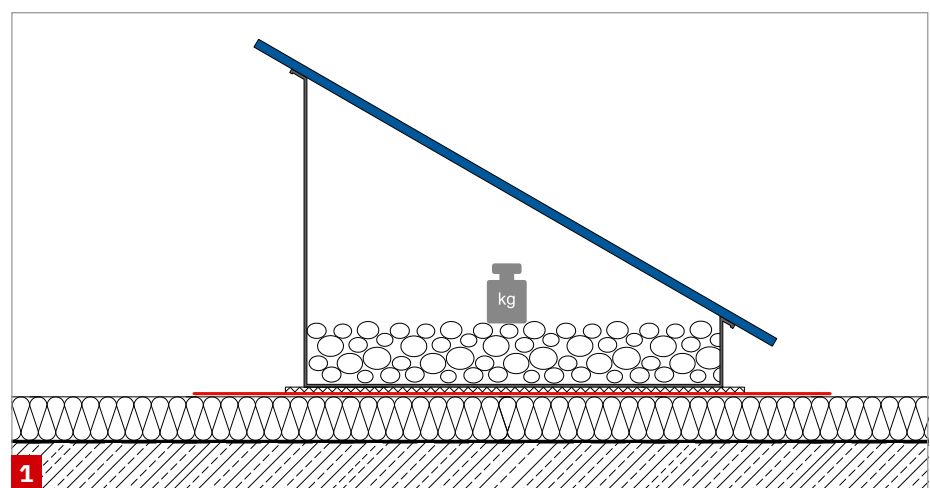
Abbildung 1: Ballastiertes System
