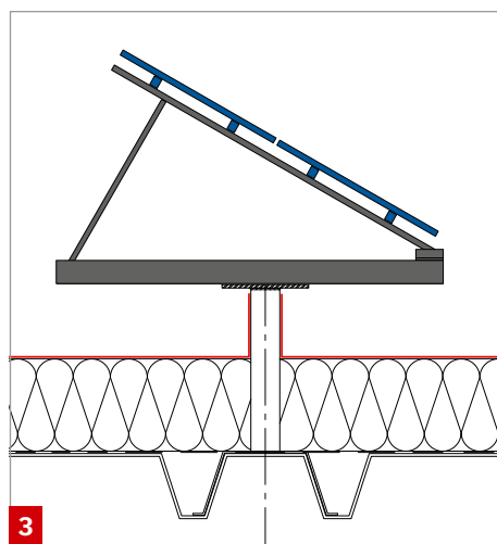
Abbildung 3: Aufgeständertes System
