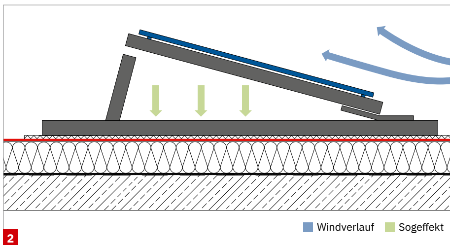
Abbildung 2: Aerodynamisches System
